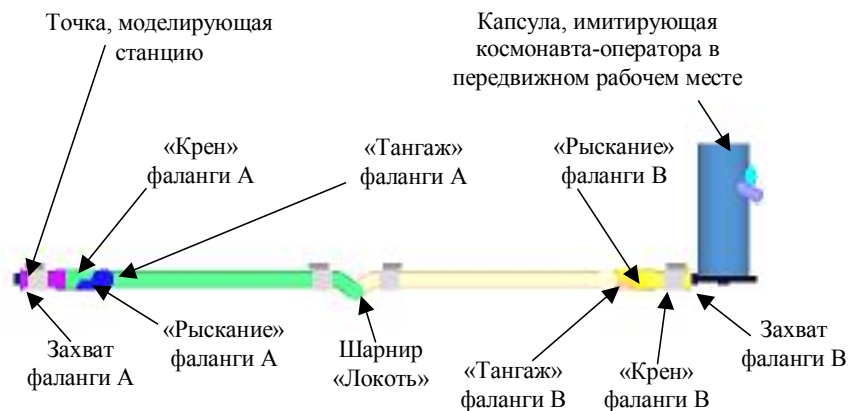
Рис.1. Внешний вид исследуемой модели конструкции «манипулятор ERA - передвижное рабочее место – космонавт», жестко закрепленной на поверхности МКС.
