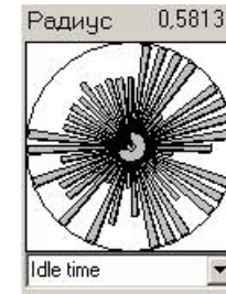
Рисунок 7. Радиальная диаграмма потери времени (простая процессоров) при выполнении программы на 78 процессорах
